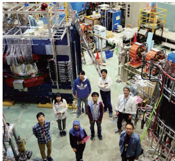
第二実験室内に設置されたNKS2実験装置（左上）。電磁石内部には標的とドリフト・チェンバーが設置されており、その周りを飛行時間測定装置が囲んでいます。右下に見えるのはメンテナンスの為に移動させた飛行時間測定装置の一部です。
