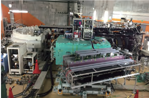
電子光物理学研究センターが理化学研究所RIビームファクトリーに設置した大型電子スペクトロメータ“WiSES: Window-frame Spectrometer for Electron Scattering”
