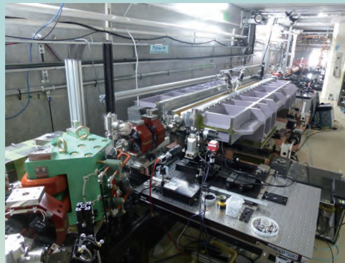
大強度電子線形加速器 1967年に建設された大強度電子加速器です。最大エネルギー：70 MeV、ビーム繰り返し：300Hz、ビームパワー：5kW以上、放射性同位元素（RI）の製造などに利用されています。
